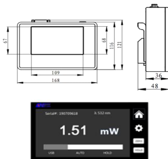
Header TP100
