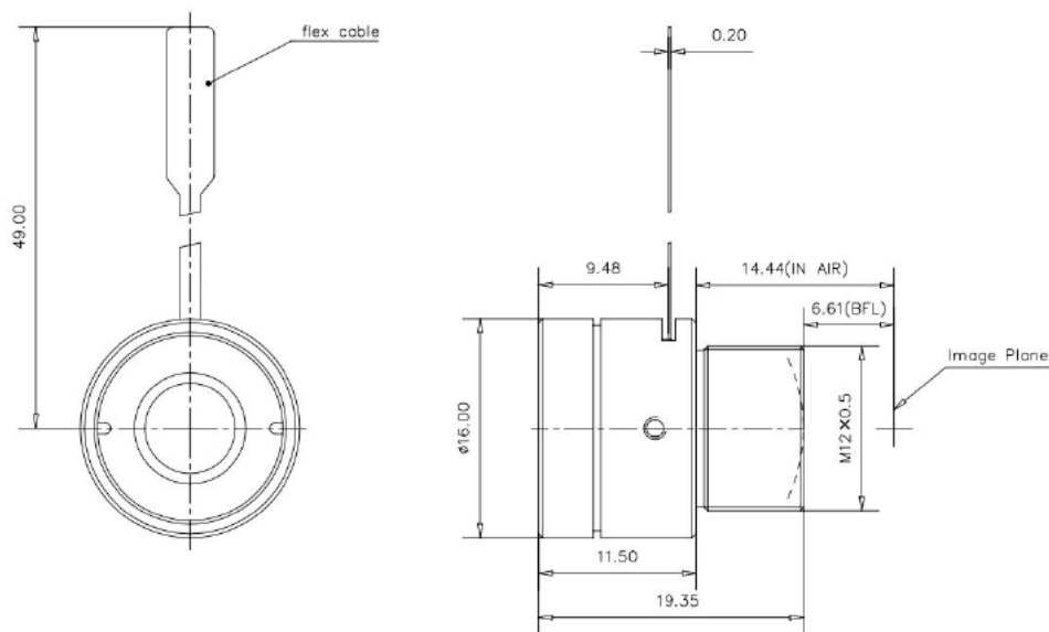
图 1：ELM-25-5.6-9-S 机械图纸
